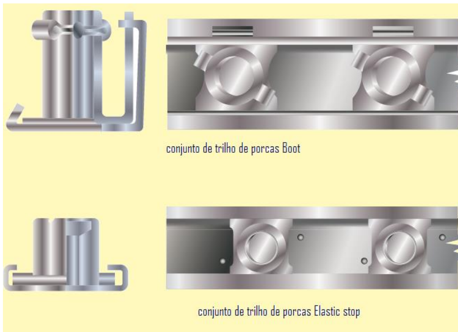
Fonte: FAA - Federal Aviation Administration - Mechanic Training Handbook Figura 6-10 - Porcas autofreno em trilhos.
