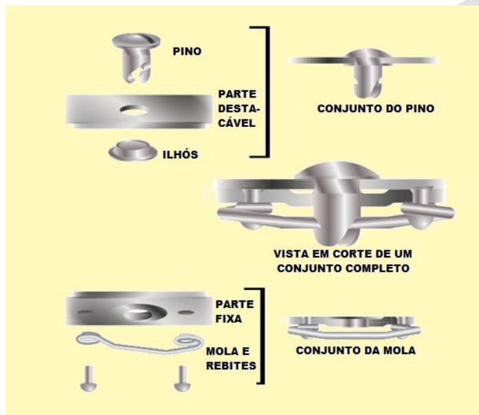
Figura 6-17 Prendedores Dzus.
