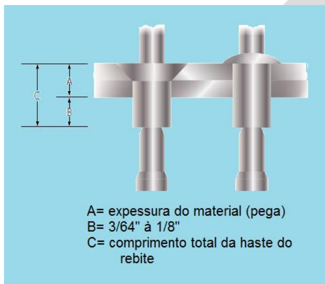
Figura 6-36 Determinação do comprimento do rebite de autocravação.
