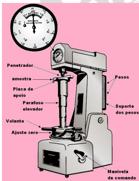
Figura 6-69 Medidor Rockwell de dureza.
